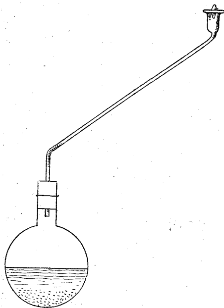
Fig. 10. — Digesteur simplifié. — Un ballon, un tubulésse terminant par un petit bouchon de verre simplement posé. Le liquide s'évapore dans les parties froides du tube et retombe; une rosace du bouchon sur la bordure du tube assure une fermeture suffisante et sans danger.
